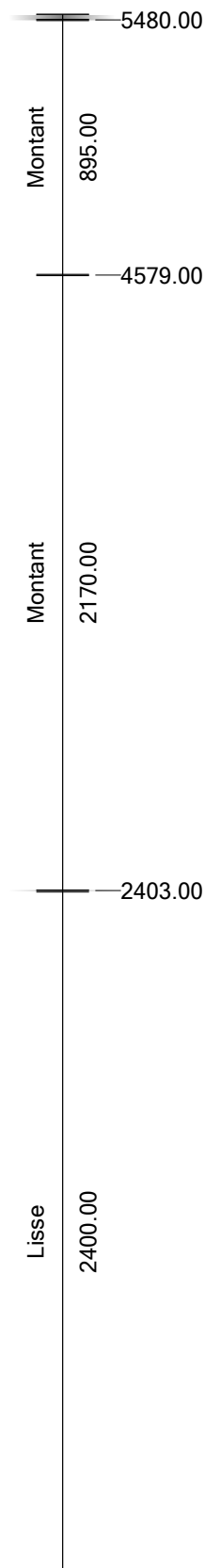
22/36 -- BM 45/145, 45.00 x 145.00 -- 5500.00 mm -- Exemple unique
