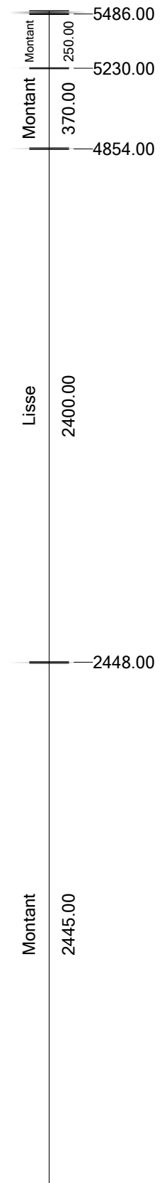
24/36 -- BM 45/145, 45.00 x 145.00 -- 5500.00 mm -- À fabriquer en 2 exemplaires
