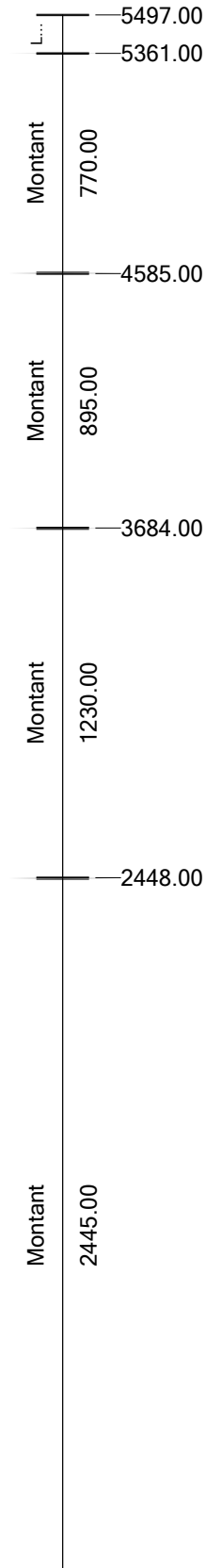
21/36 -- BM 45/145, 45.00 x 145.00 -- 5500.00 mm -- Exemple unique
