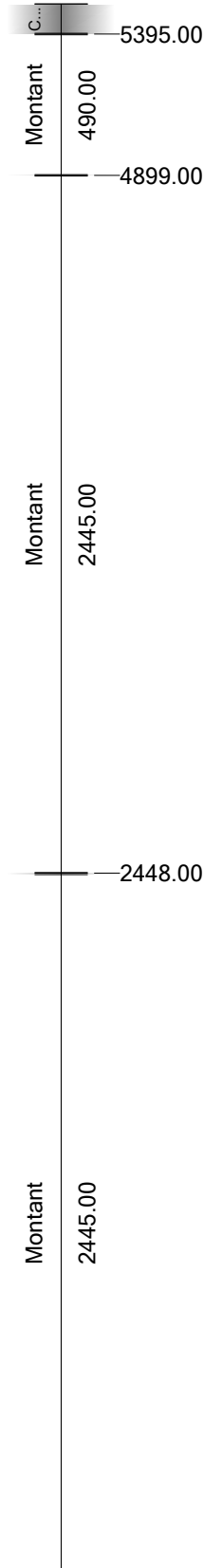
31/36 -- BM 45/145, 45.00 x 145.00 -- 5500.00 mm -- À fabriquer en 3 exemplaires
